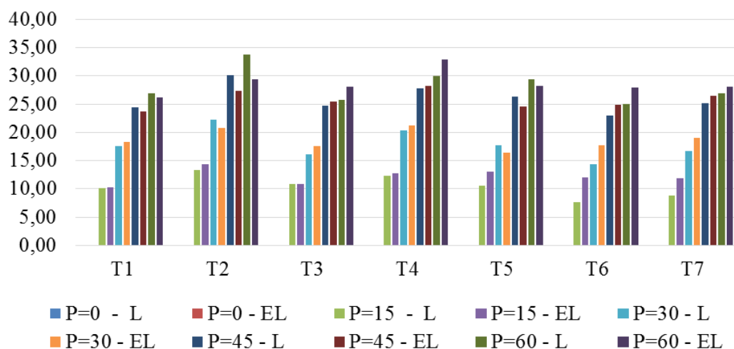
Figura 2: Resistência mecânica do solo à penetração na área experimental da Fazenda de Ensino, Pesquisa e Extensão da UNESP, Campus de Ilha Solteira, localizada no município de Selvíria-MS (2012/13).
